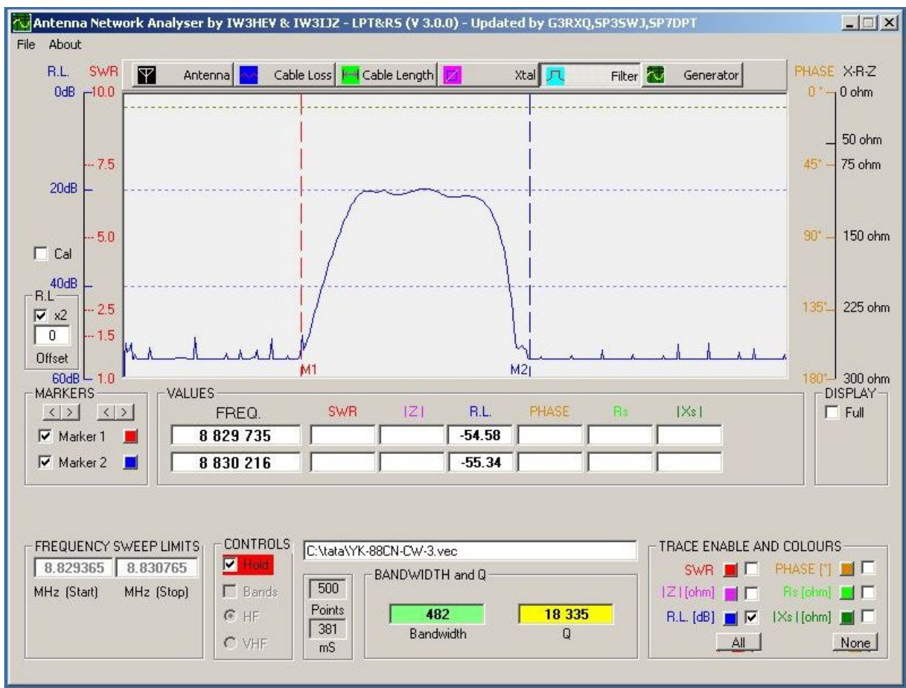
Filtr kwarcowy firmy Kenwood YK-88CN-CW
