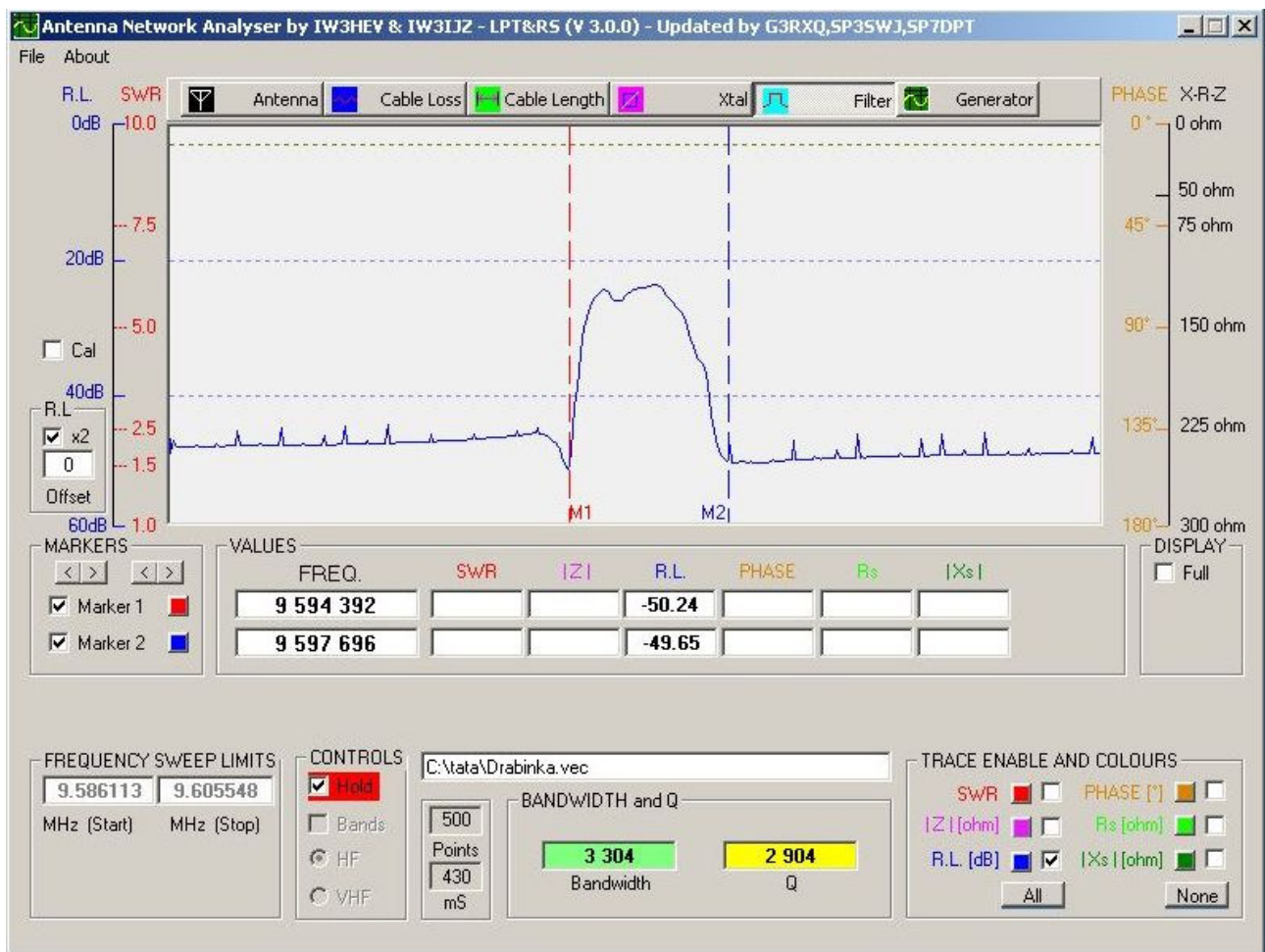
Filtr drabinkowy 6- kwarcowy amatorski
