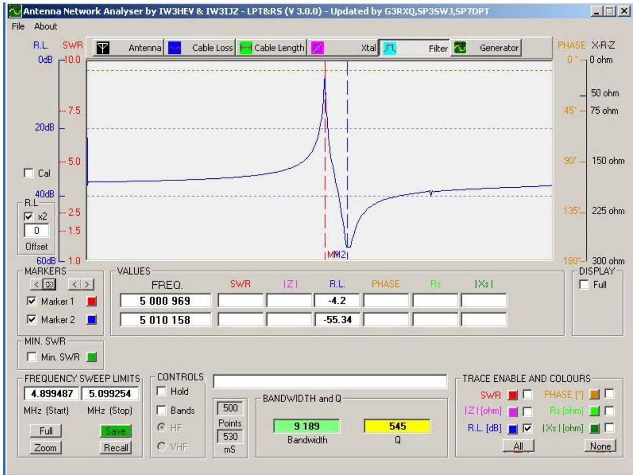
Pomiar kwarcu 5MHz
